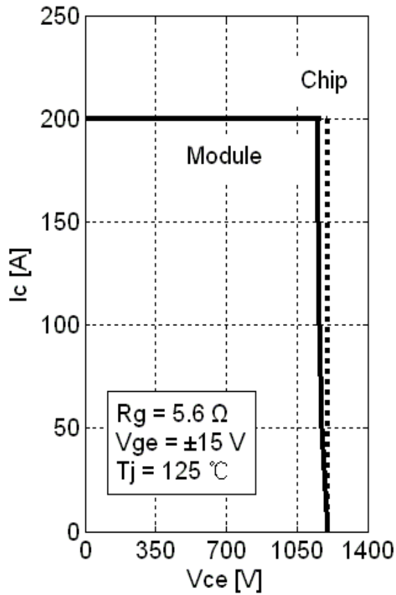
Fig 5. RBSOA
